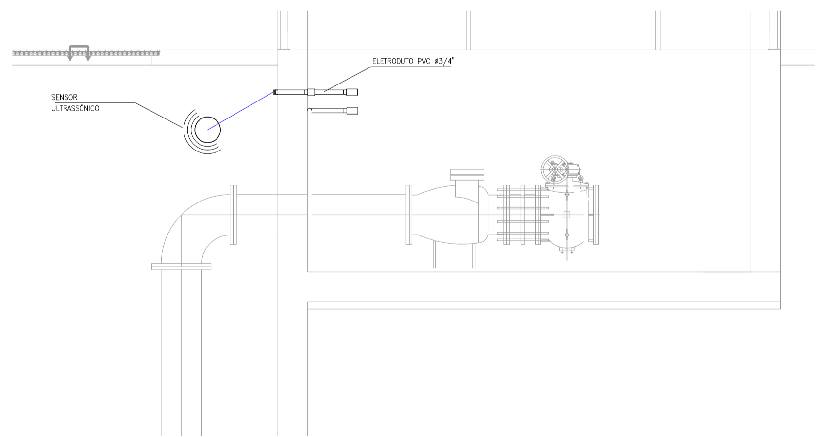
2 DETALHE LIGAÇÃO DO SENSOR ULTRASSONICO ESCALA 1/25
